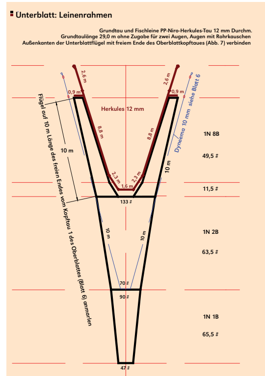
Abbildung 9: Leinenrahmen des Unterblattes vom reduzierten Grundschleppnetz.
