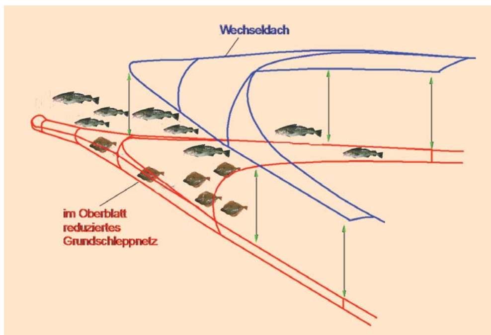
Abbildung 13: Funktionsprinzip des reduzierten Grundschleppnetzes mit Wechseldach.
