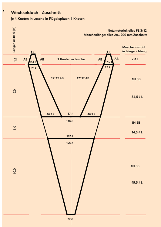
Abbildung 10: Zuschnitt des Wechseldaches für das Topless-Trawl.
