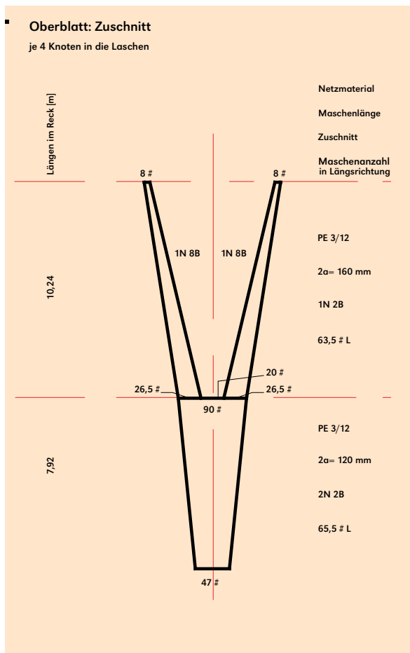
Abbildung 6: Zuschnitt des reduzierten Oberblattes.
