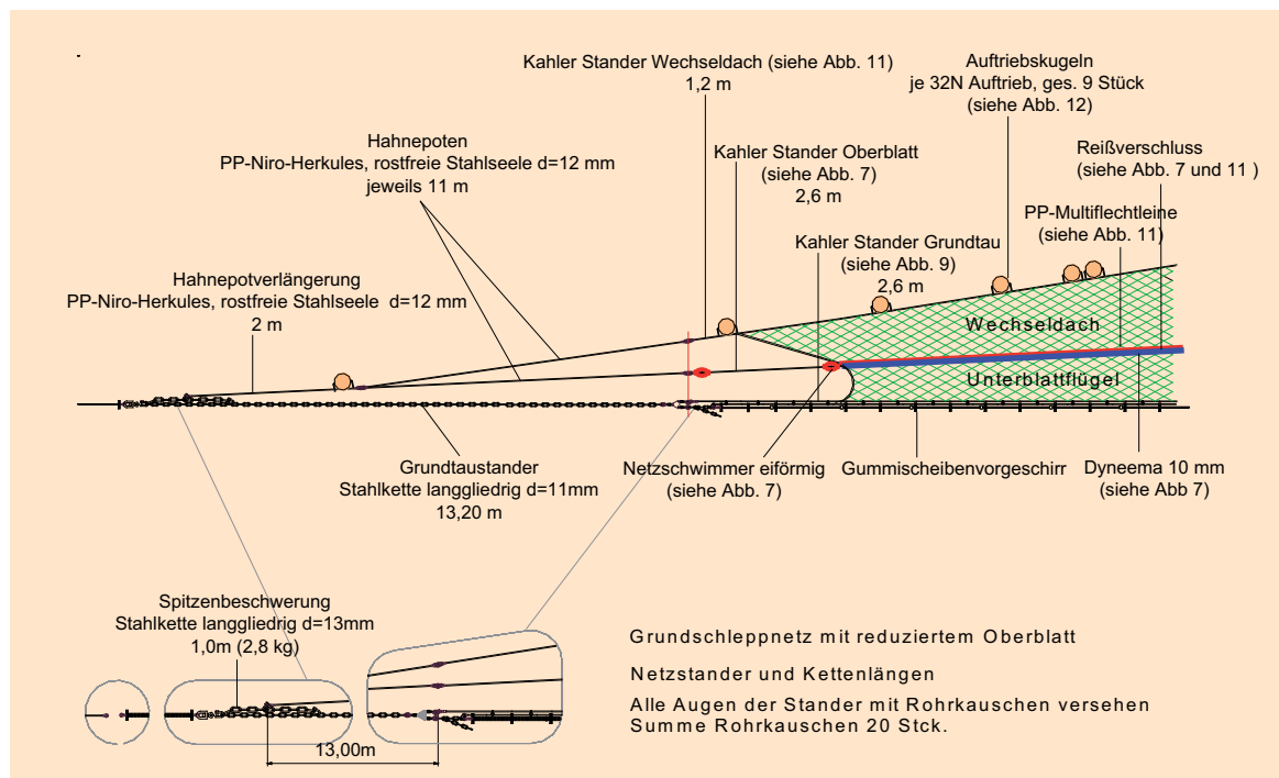
Abbildung 14: Netzstander des reduzierten Grundschieppnetzes mit Wechseldach.
